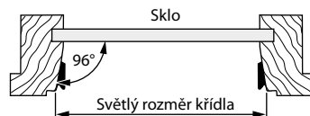
Typ křídla A
